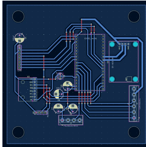
Figura 24: Diseño PCB de Cortex.
