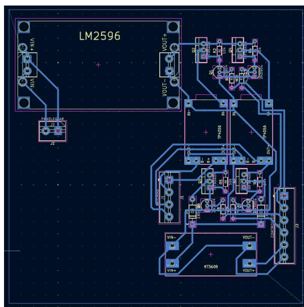
Figura 10: Circuito PCB de Solaria.
