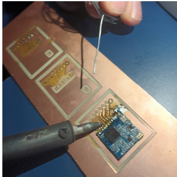
Figura 16: Proceso de soldado de módulo LoRa.
